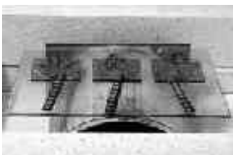
Biegeform in der Anwendung / Forming with a mold
